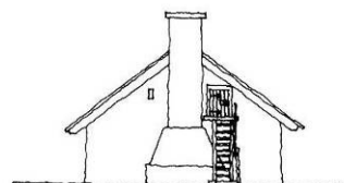
DÉLNYUGATI HOMLOKZAT
